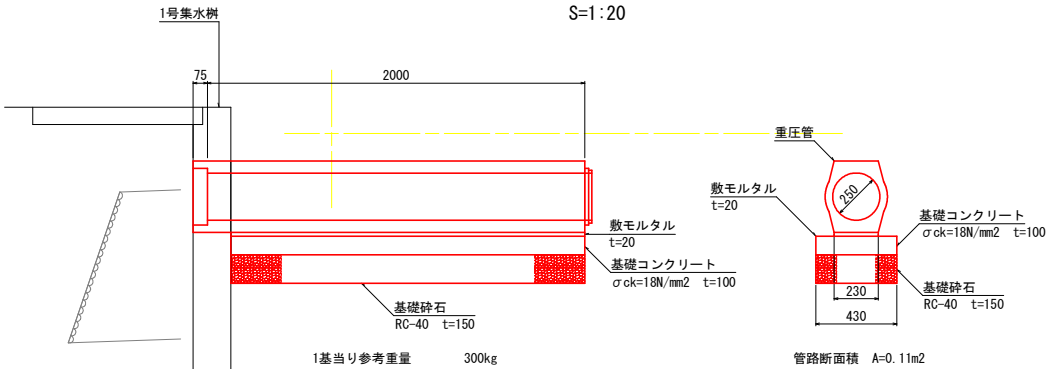
管路復旧工
