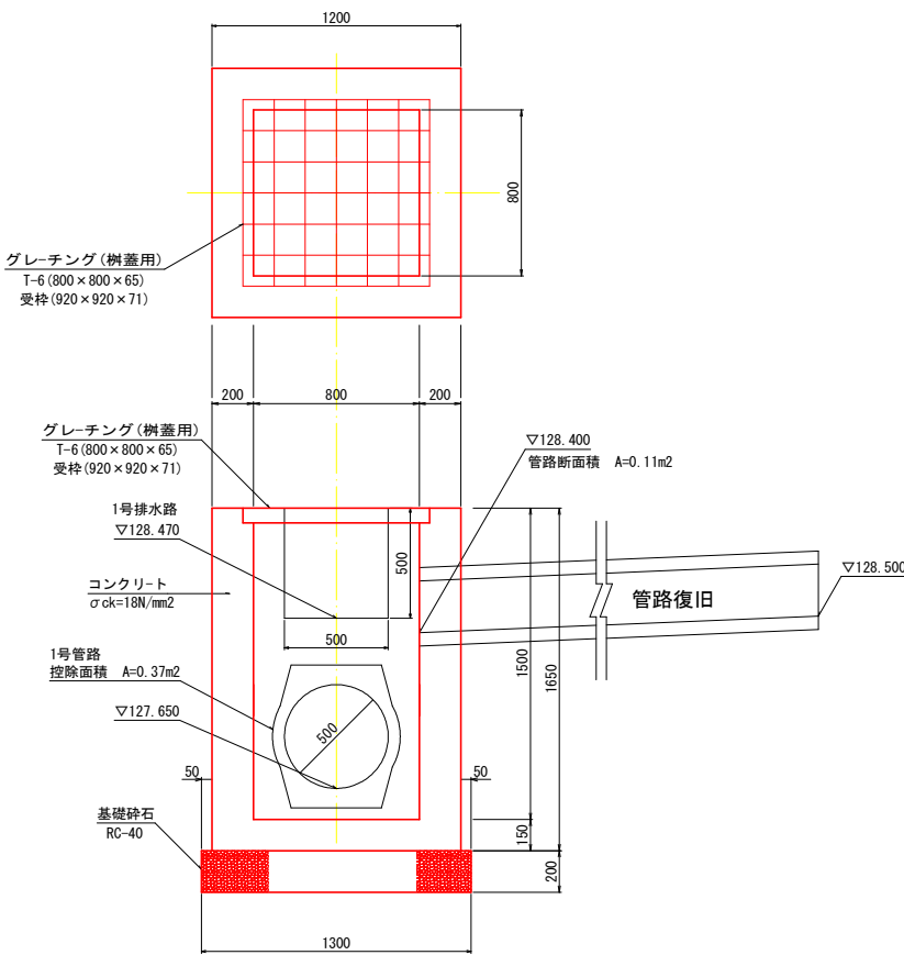
1号集水樹
