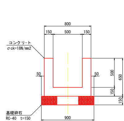
1号排水路工
