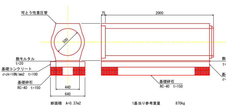
1号管路工
